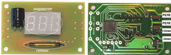
Рисунок 1. Таймер-счетчик. Общий вид.
