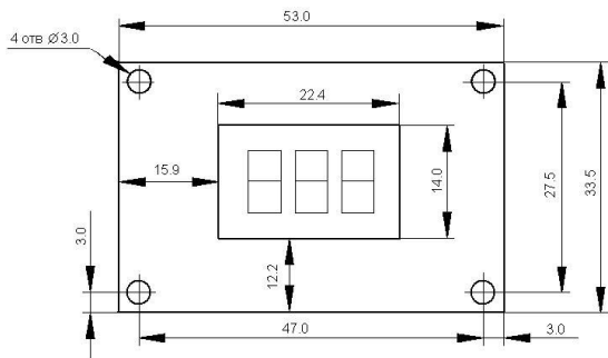
Рисунок 2. Таймер-счетчик. Габаритные и монтажные размеры.
