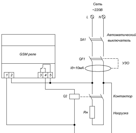
Рисунок 4. Схема включения нагрузки больше 16А.
