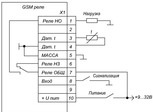
Рисунок 3. Типовая схема включения GSM реле.
