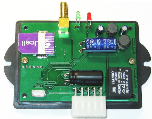
Рисунок 2. Установка SIM карты.
