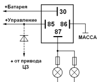
Рисунок 1. Реле защиты ламп.
